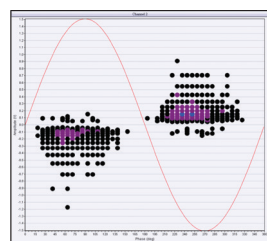
Resolución de fase 2D
