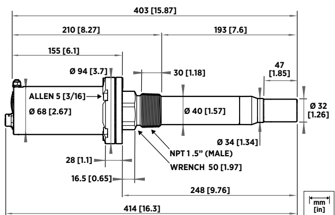
MGP262 dimensions
