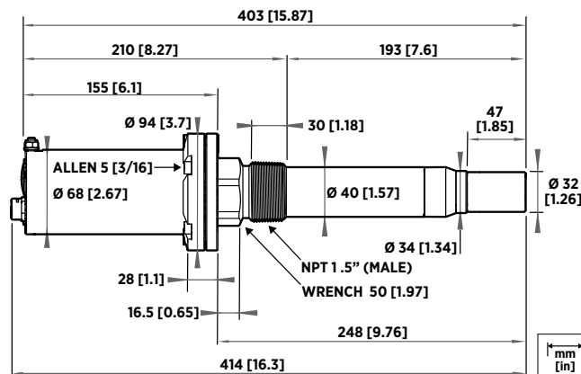
MGP261 dimensions
